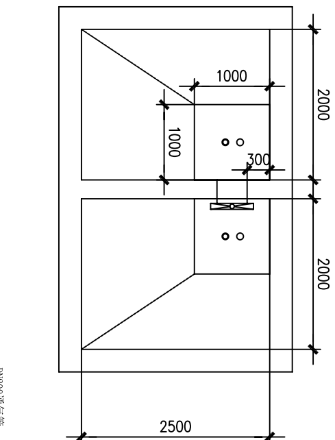
下层平面图
