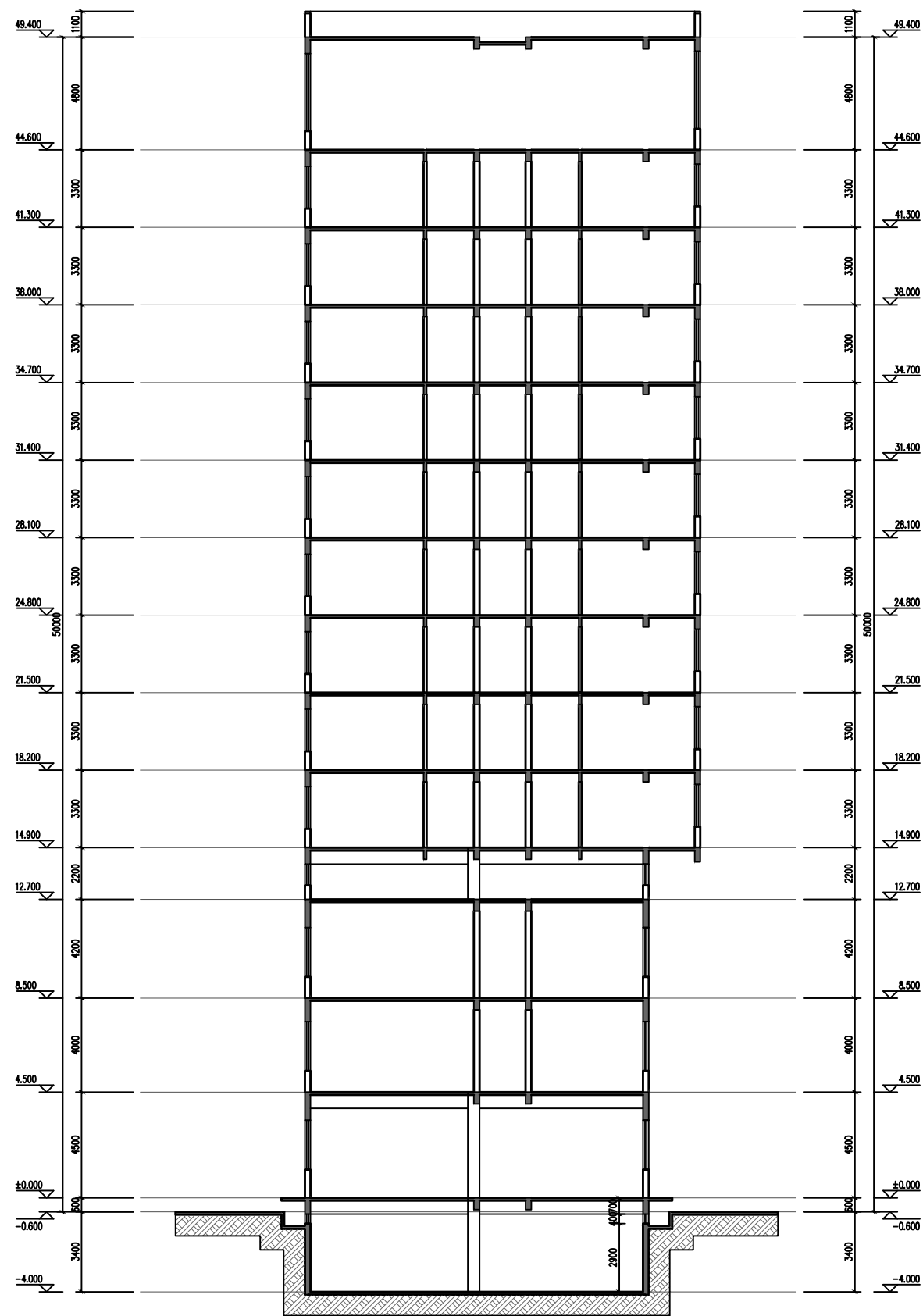
1-1剖面图
